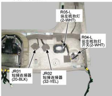
220.车顶装饰板前左
