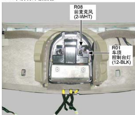
221.车顶装饰板前部
